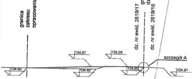
PRZEKRÓJ T1-T1
