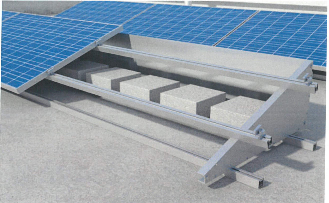
Przykład montażu paneli na dachu płaskim z wykorzystaniem konstrukcji wsporczej balastowanej
